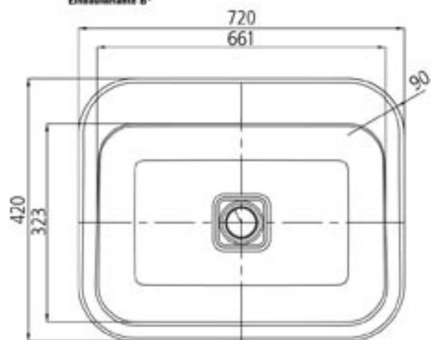
Einbauvariante B*
