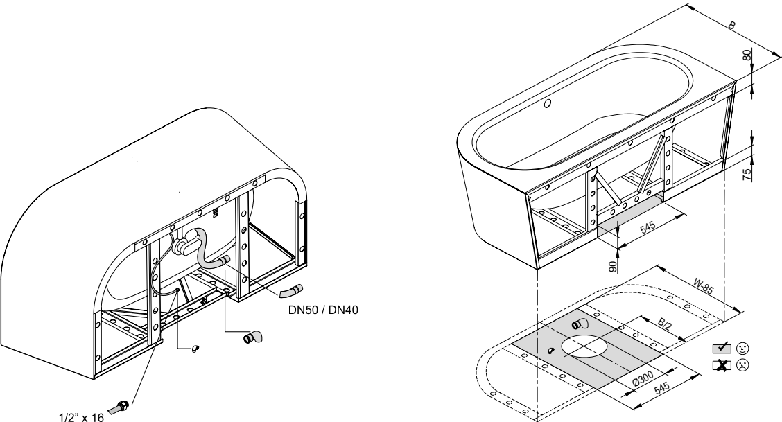
Anschlussmaße für Ab- und Überlaufgarnitur
